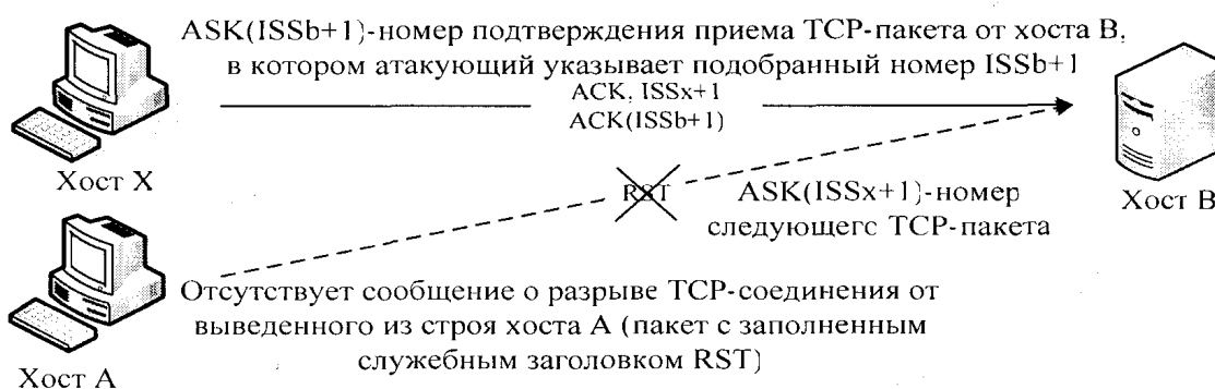
"Рисунок 7. Схема реализации угрозы "Подмена доверенного объекта сети"
