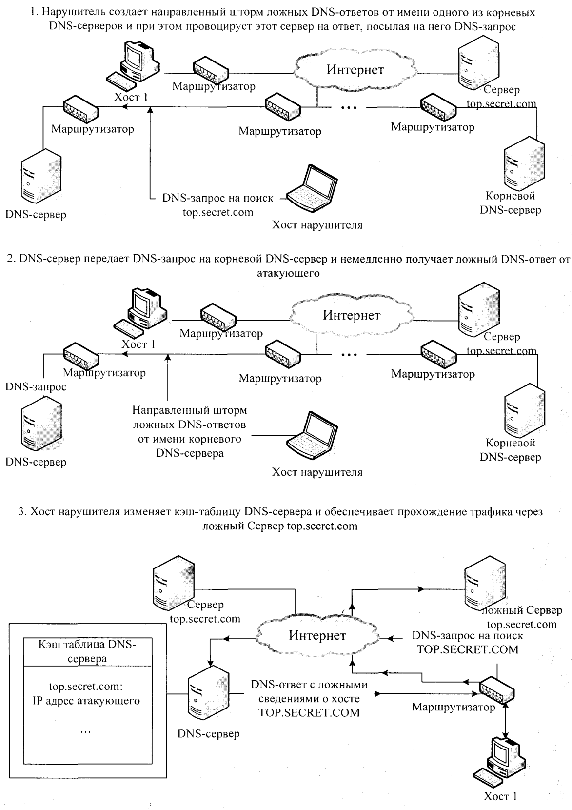
исунок 13. Схема реализации угрозы "Внедрение ложного DNS-сервера" путем шторма DNS-ответов на DNS-сервер"
